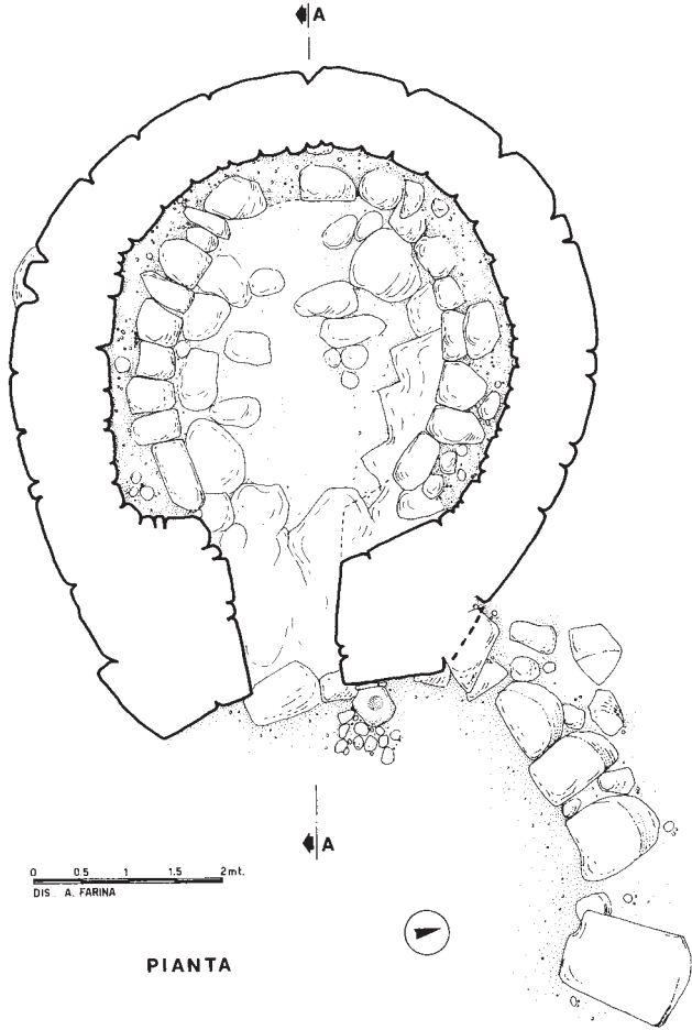
Fig. 41 Capanna 49: pianta e sezione.
