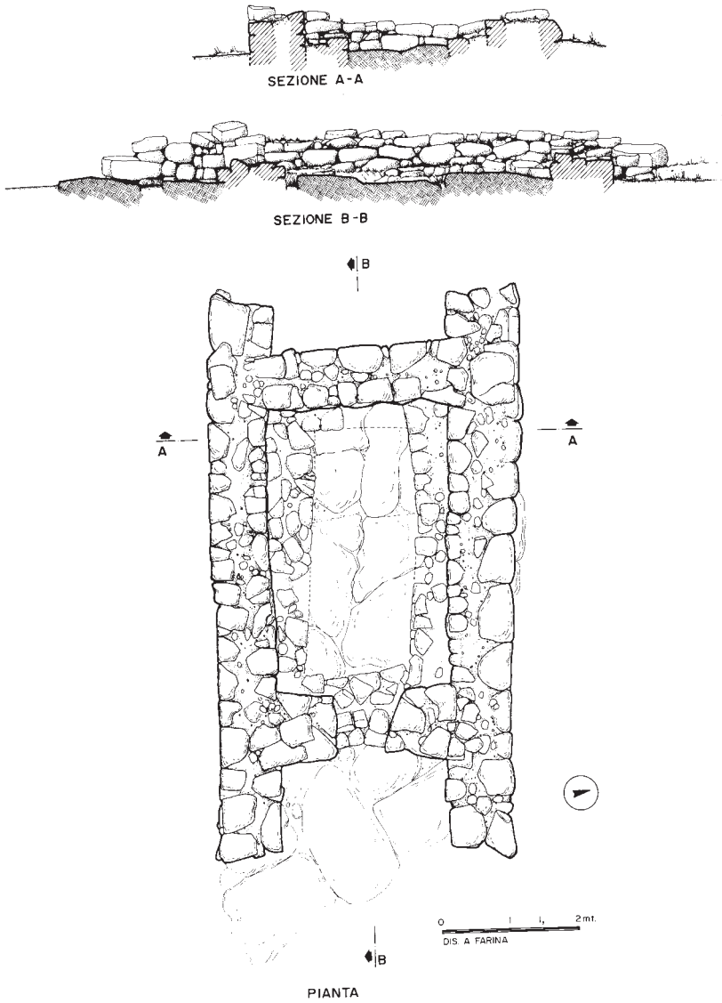
Fig. 46 Tempio A: pianta e sezione.
