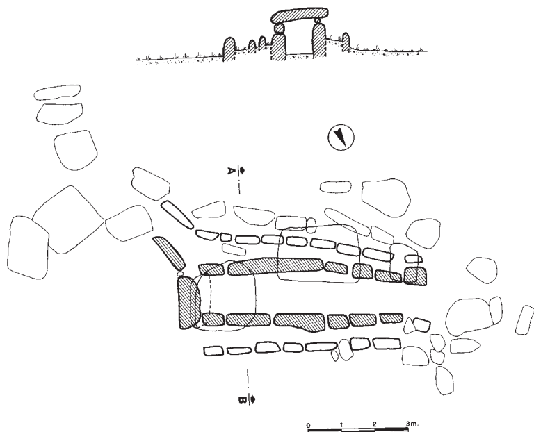
Fig. 20 Tomba di giganti Su Barcu I: pianta e sezioni.
