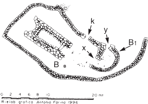
Fig. 49 Planimetria del Recinto B con Tempietto e Vano B1.
