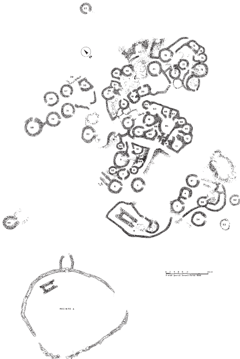
Fig. 25 Complesso nuragico di Serra Orrios: planimetria generale.
