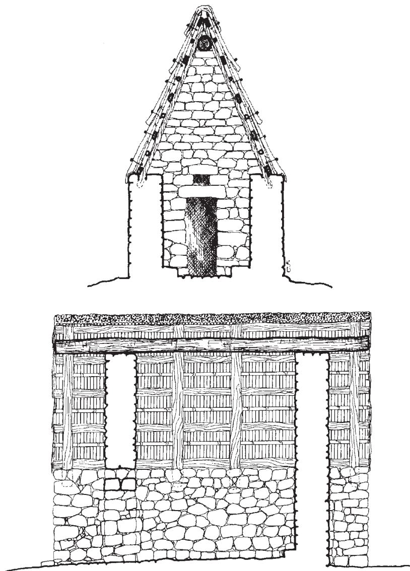
Fig. 57 Ipotesi ricostruttiva dei Tempietti a megara di Serra Orrios: prospetto e pareti laterali.
