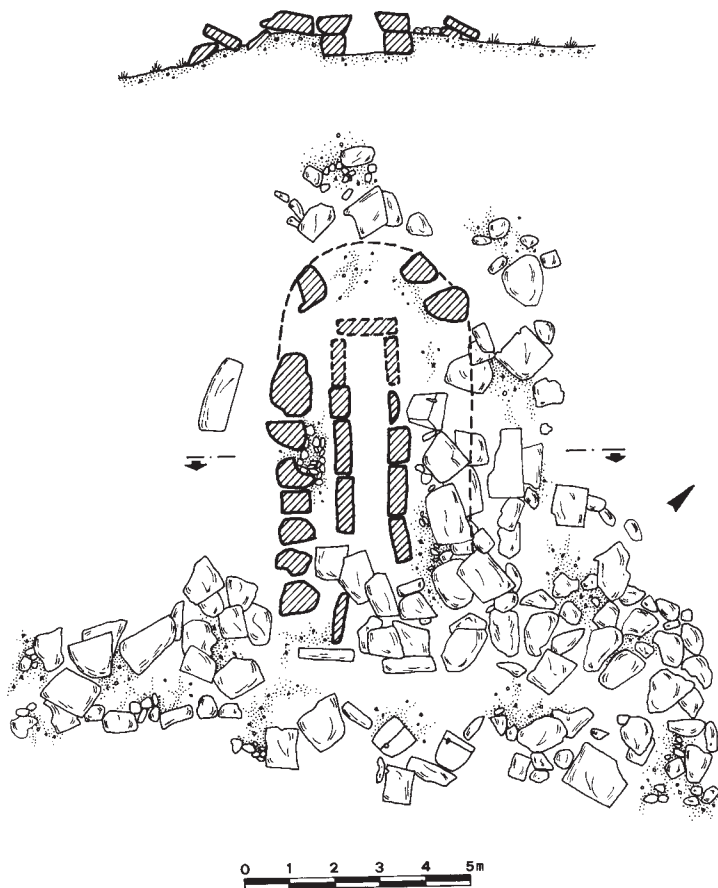
70 Tomba di giganti di Biristeddi II: planimetria.
