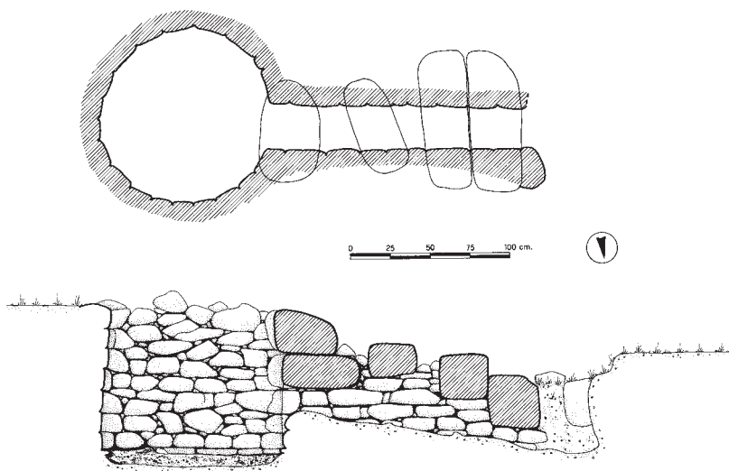
Fig. 24 Pozzo sacro (?), nuragico, di Sorgolitta: panta e sezione.
