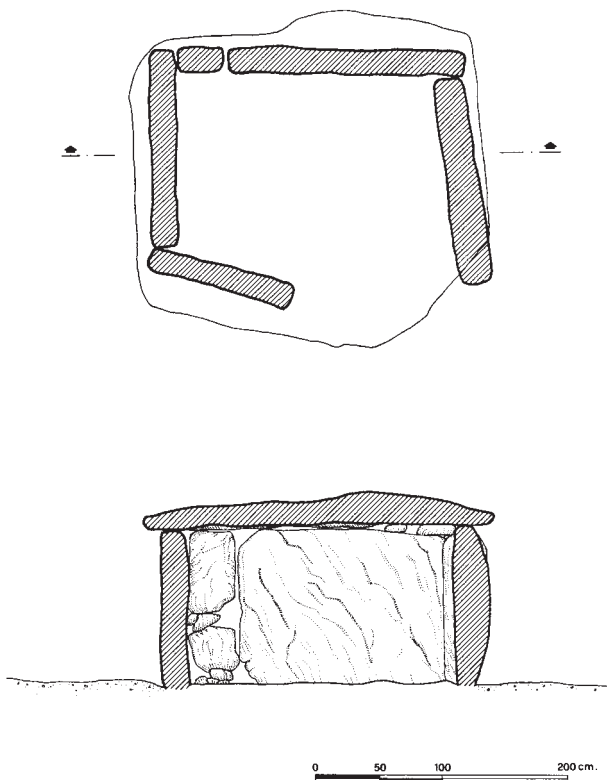
Fig. 81 Dolmen di Monte Longu: pianta e sezione.
