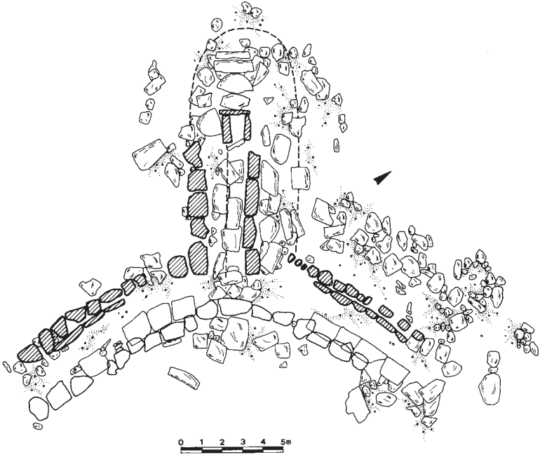
Fig. 69 Tomba di giganti di Biristeddi I: planimetria in un rilievo del 1980.
