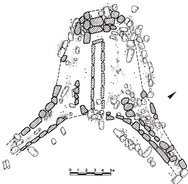
Fig. 72 Tomba di giganti di Biristeddi III: planimetria.
