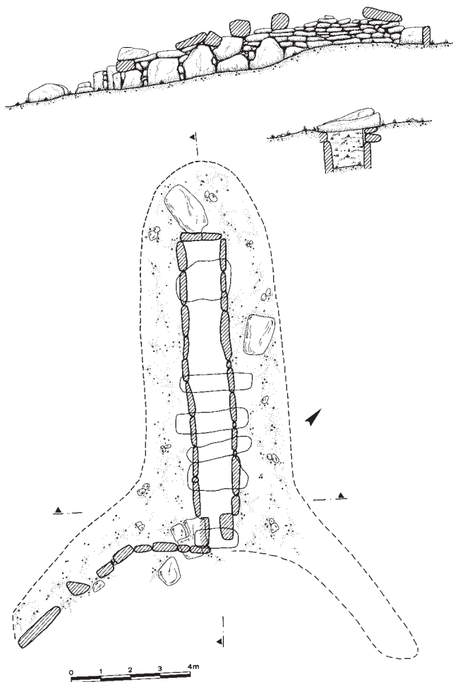
Fig. 21 Tomba di giganti di Sueredu: pianta e sezione.
