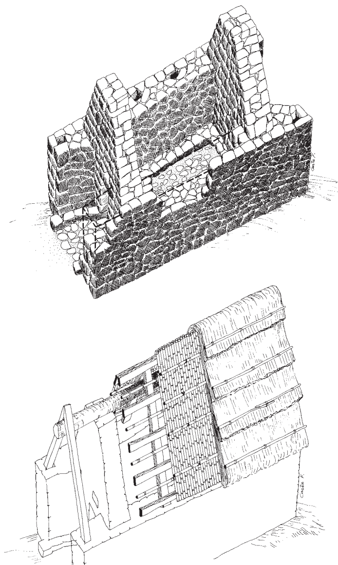
Fig. 56 Ipotesi ricostruttiva del tetto a doppio spiovente dei Tempietti a megara di Serra Orrios.
