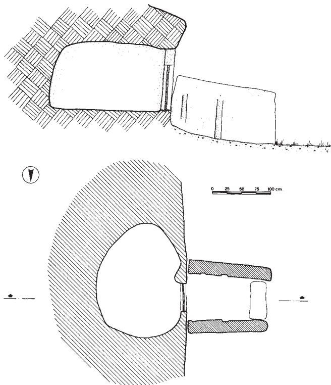
Fig. 7 Pianta e sezione della tomba ipogeico-megalitica di Mariuglia.
