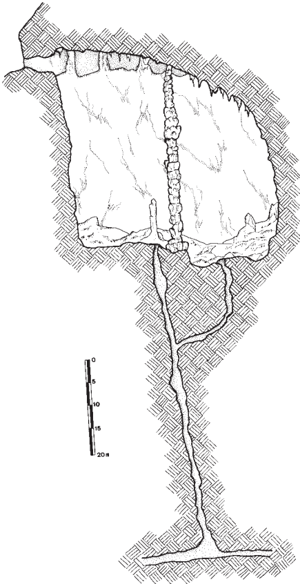
Fig. 75 Voragine di Ispinigoli: sezione.
