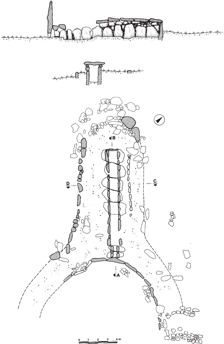
Fig. 62 Tomba di giganti di Thomes: pianta e sezioni.
