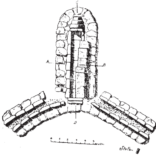
Fig. 68 Tomba di giganti di Biristeddi I: planimetria nel rilievo del Taramelli.
